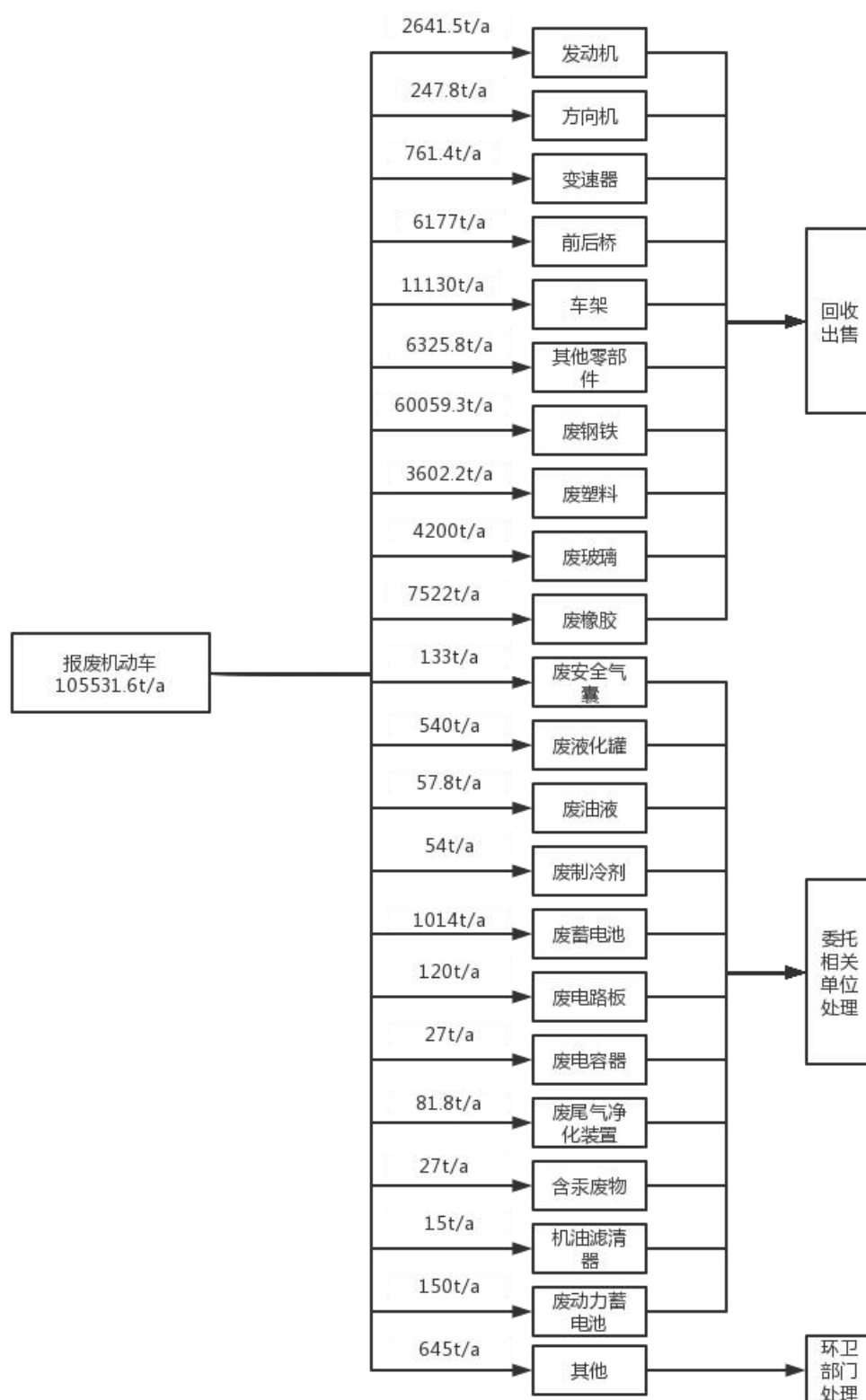
图 2-1 项目物料平衡图
