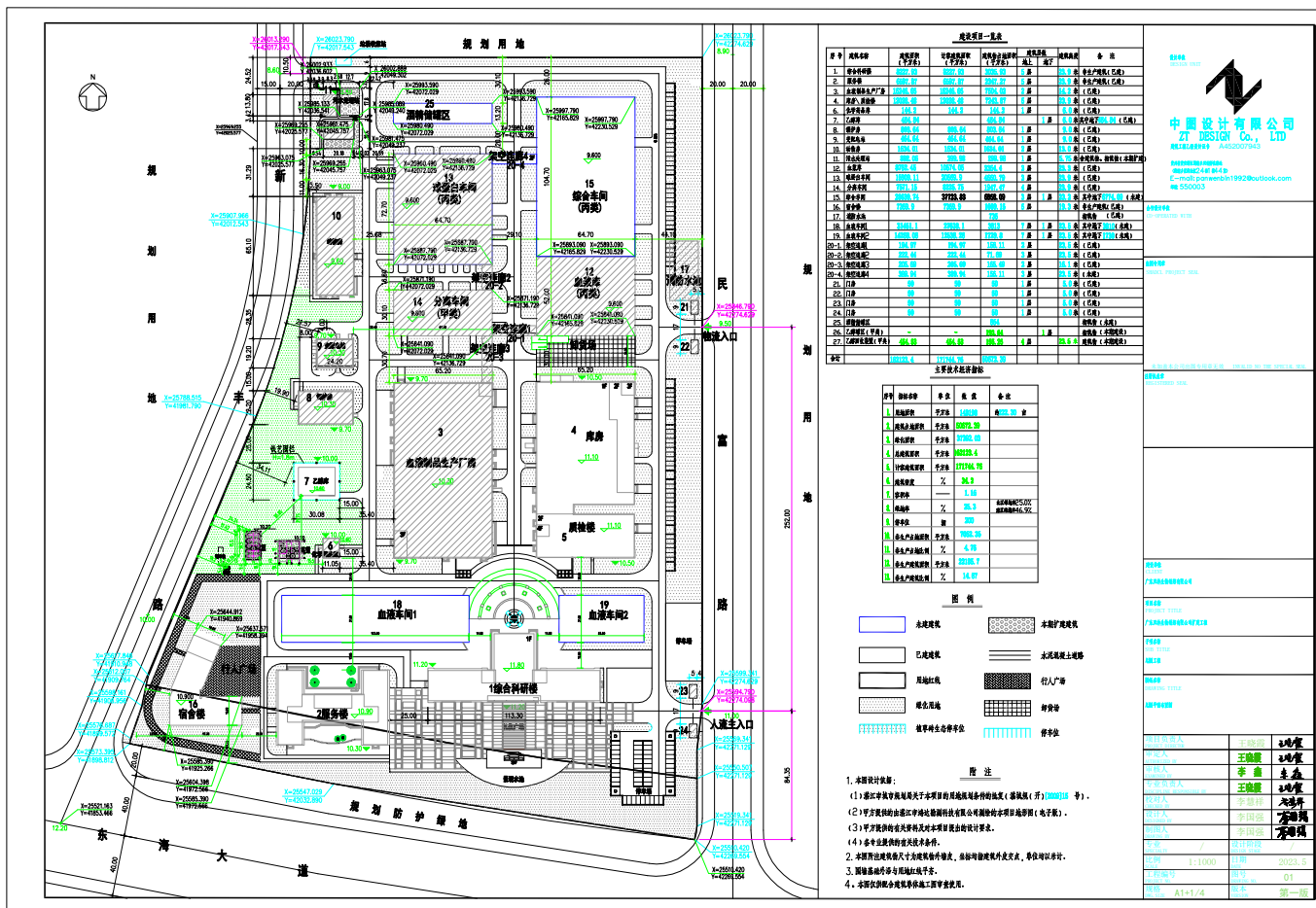
总平面图
