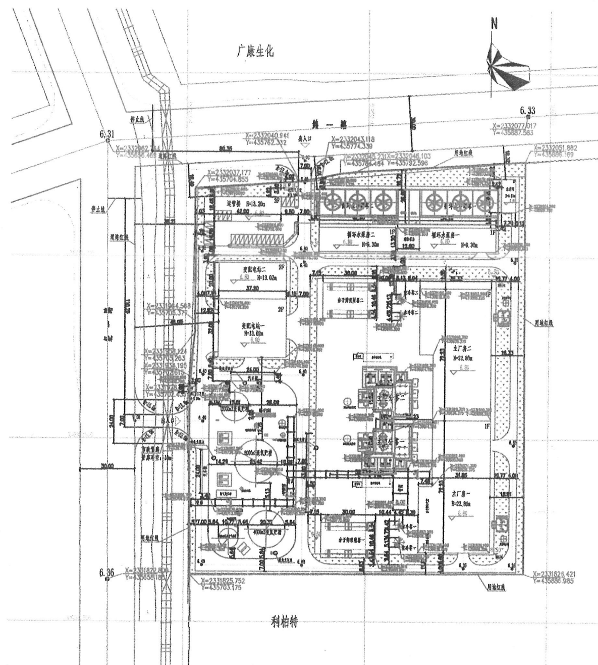
规划总平面图
