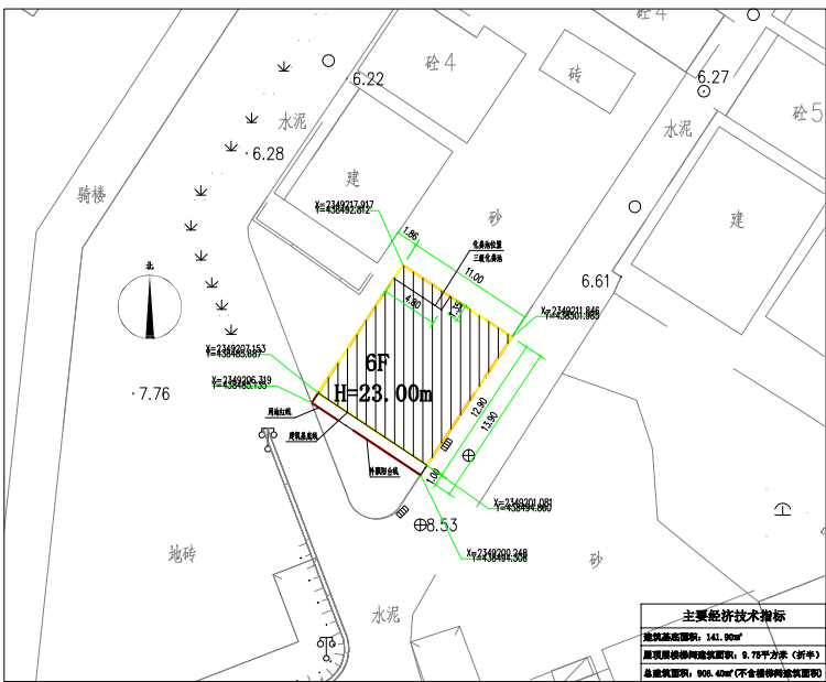
总平面图
