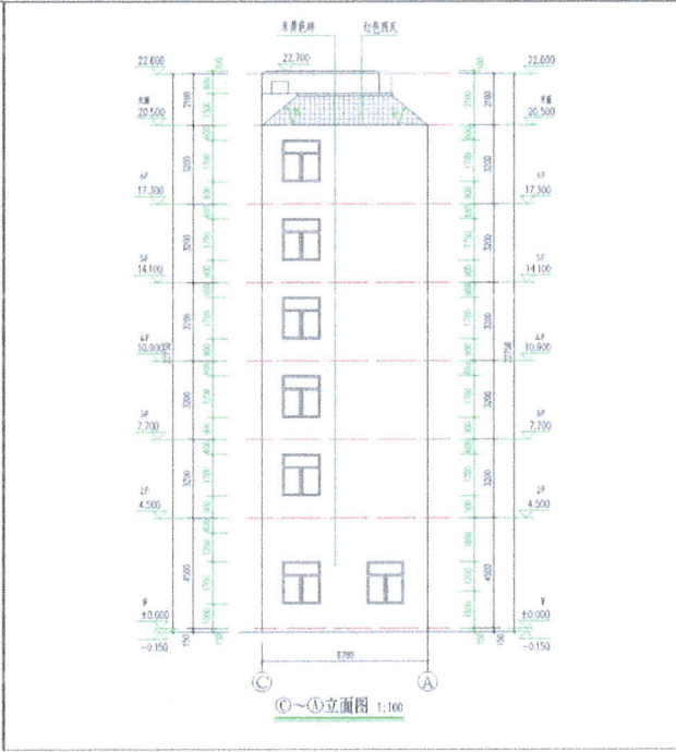
(北立面图)
