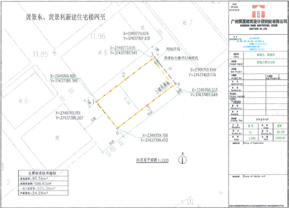
(总平面)
