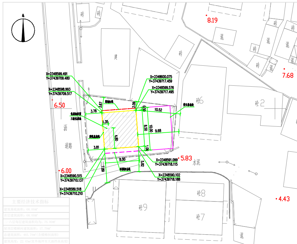
总平面图
