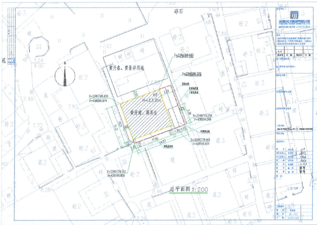
（总平面图）
