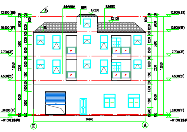
E~A轴立面图
