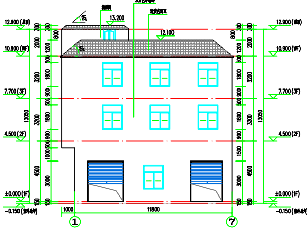
1~7轴立面图
