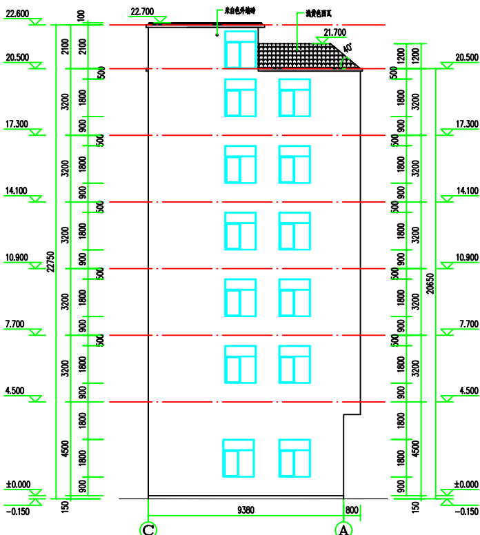
C~A 立面图
