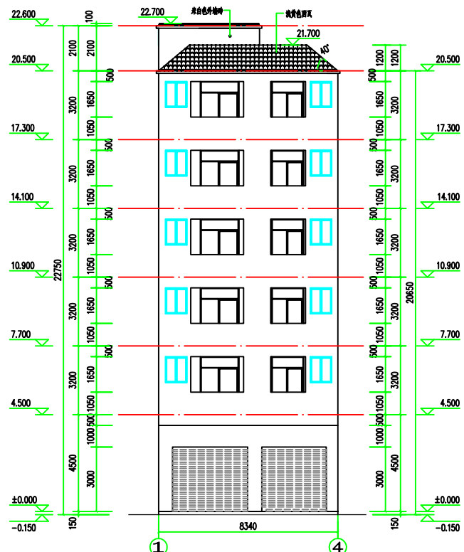
①~④ 立面图
