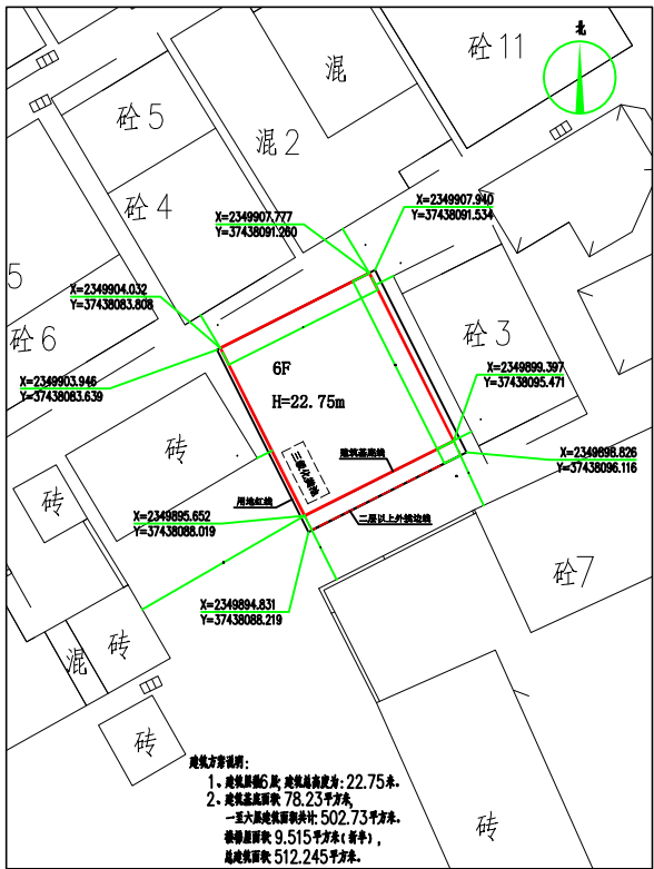
总平面图
