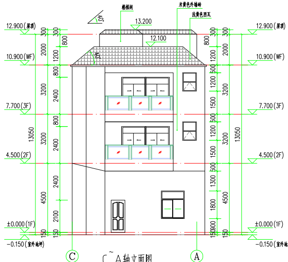
C~A轴立面图
