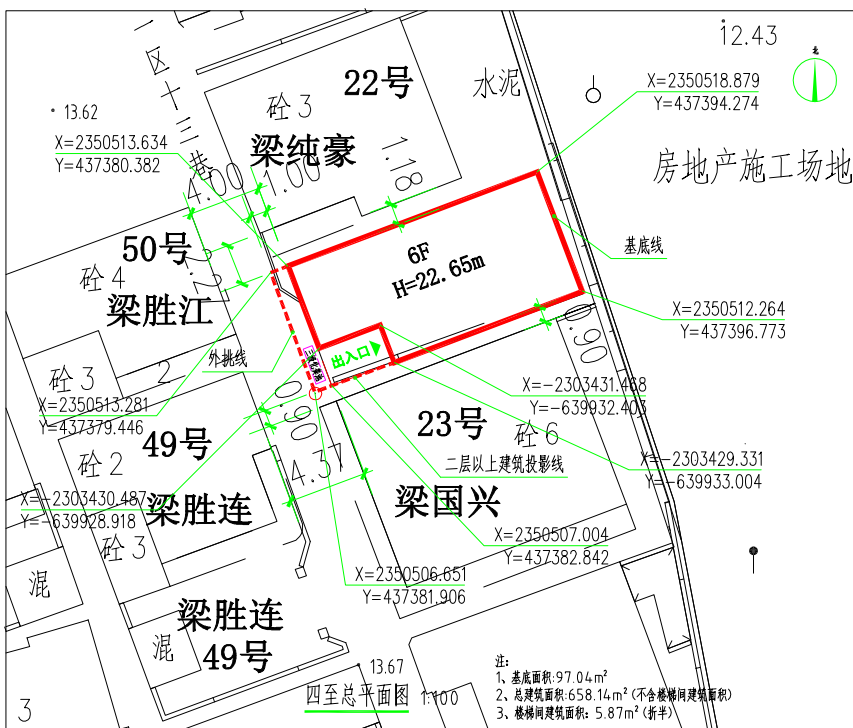
四至总平面图
