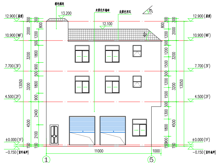
1~5轴立面图
