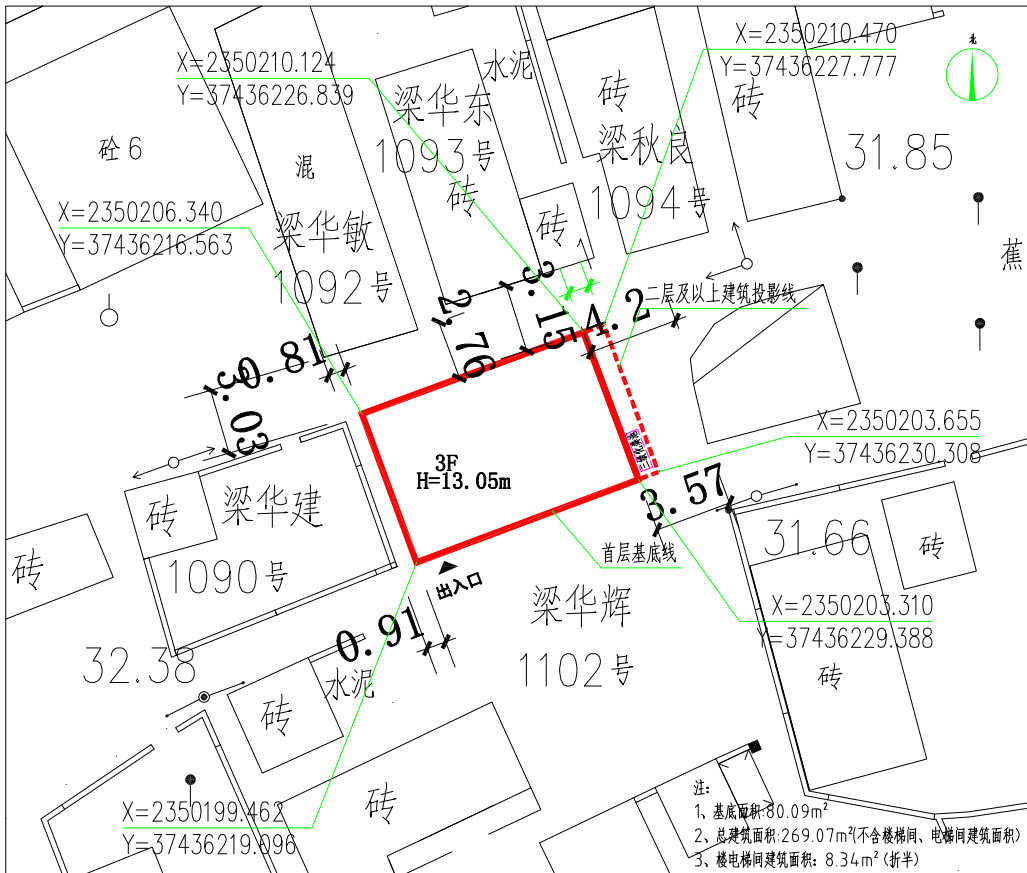
四至总平面图
