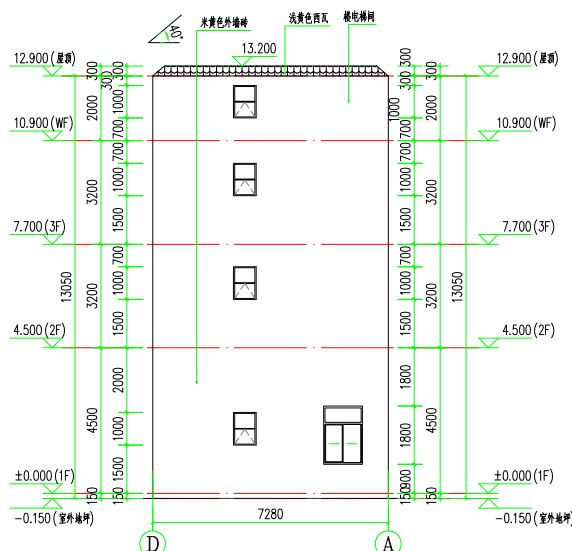
D~A轴立面图
