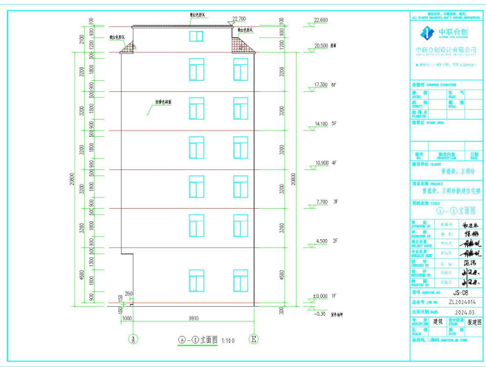
（东立面图）
