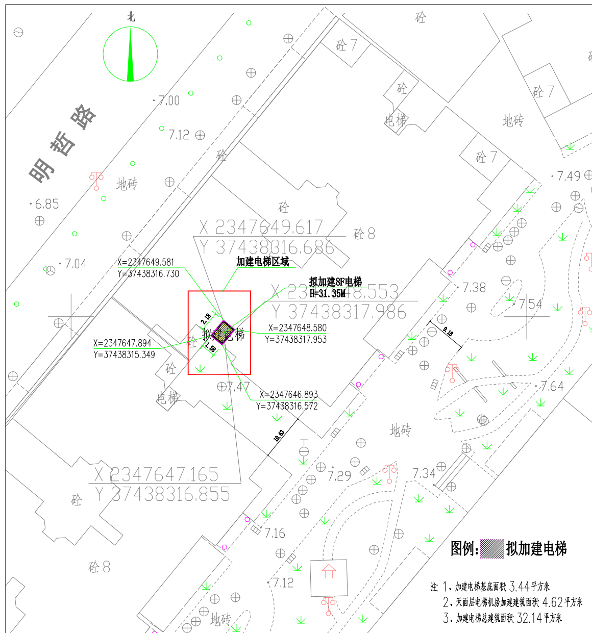
总平面图
