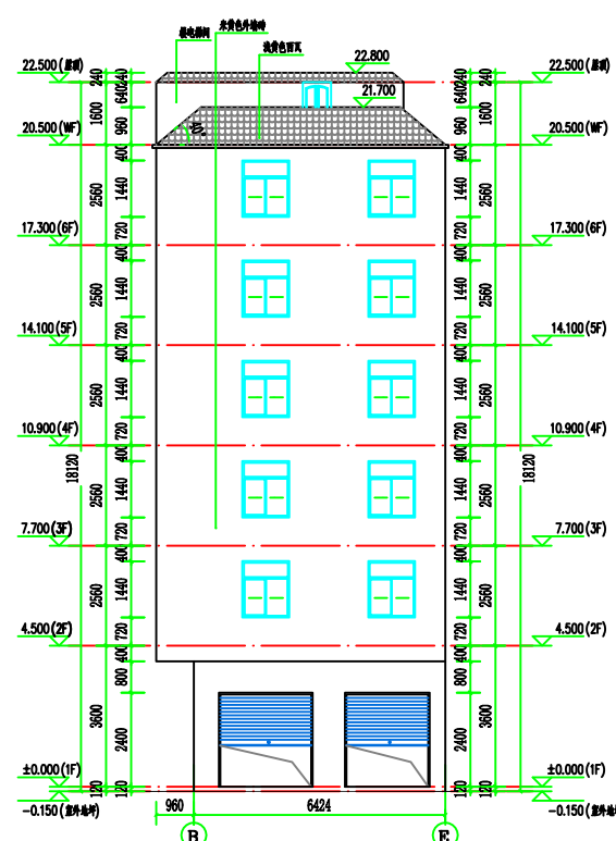
B~E 轴立面图 1:100
