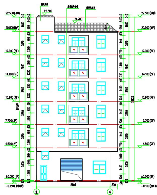
1~4 轴立面图 1:100
