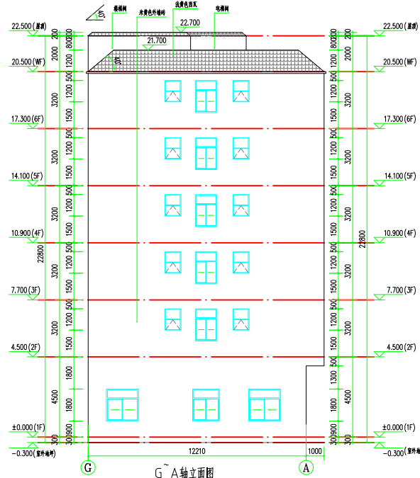
G~A轴立面图
