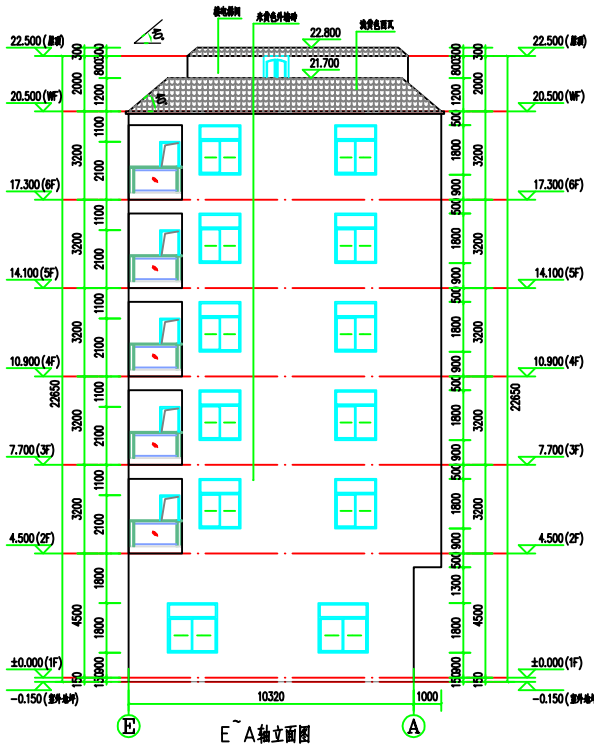
E~A轴立面图
