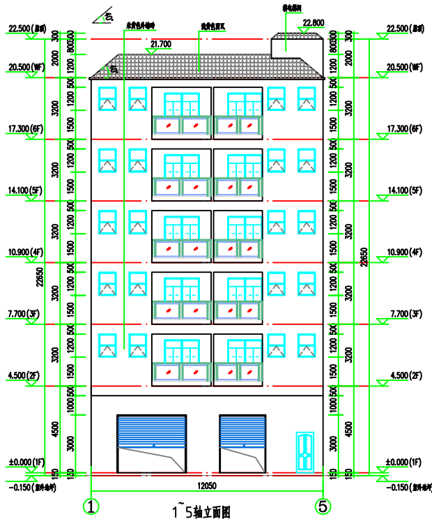
1~5轴立面图
