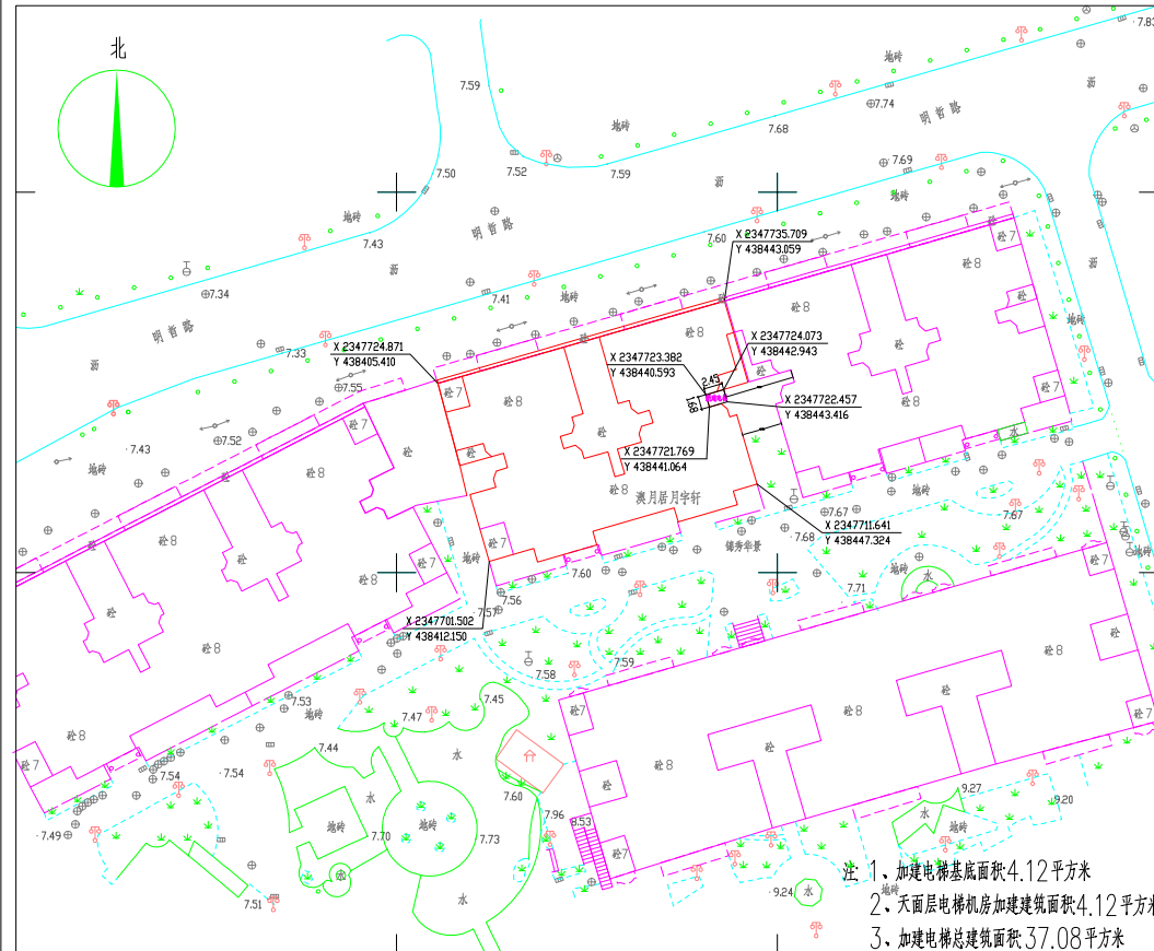
总平面图
