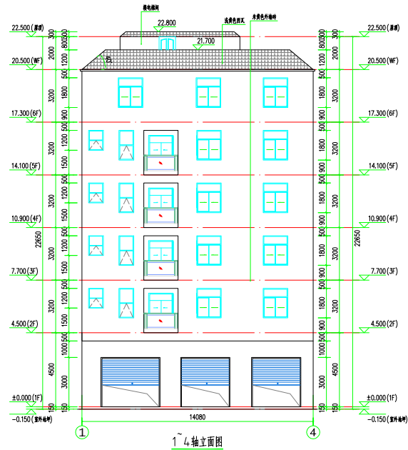
1~4轴立面图
