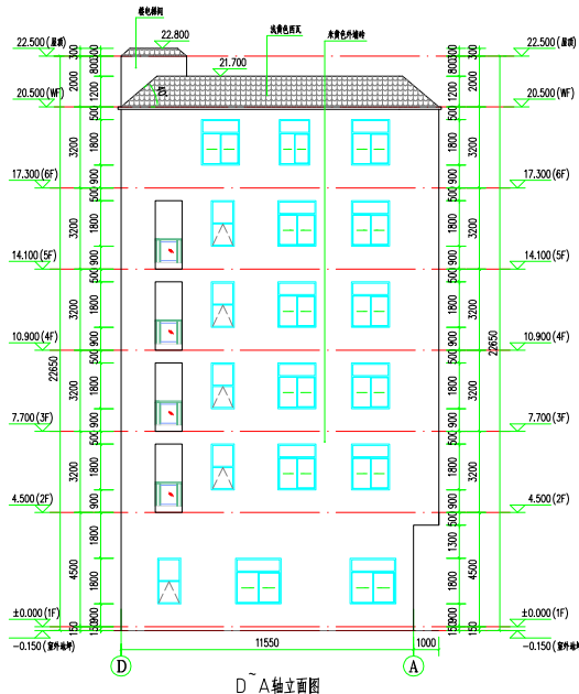
D~A轴立面图
