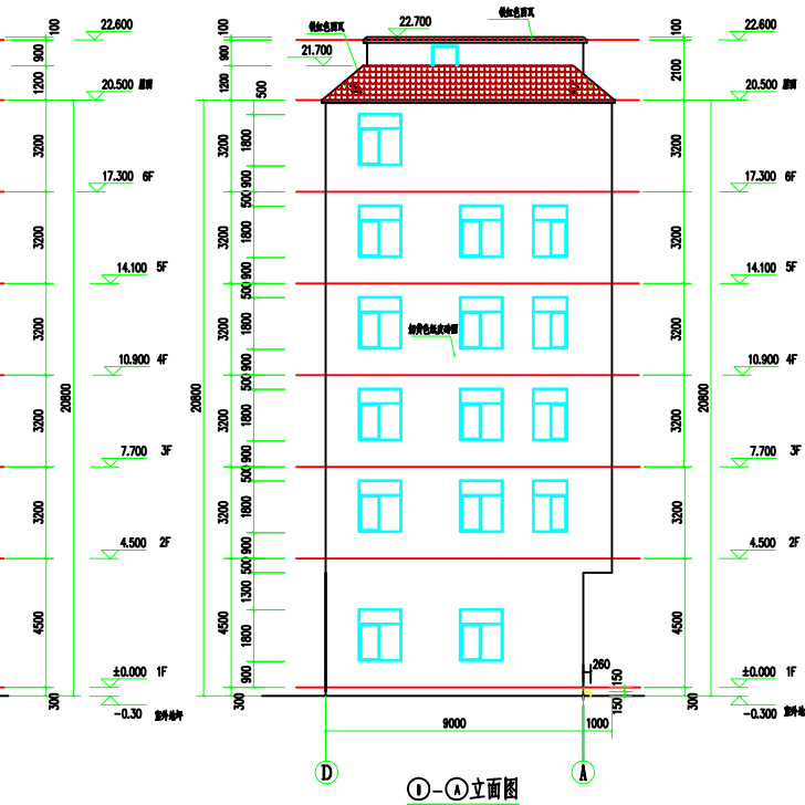
①-A立面图
