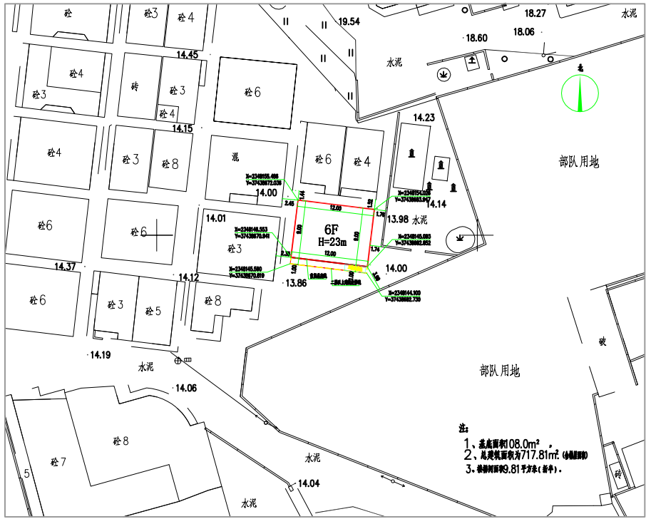
四至总平面图
