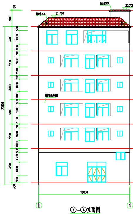
①-④立面图
