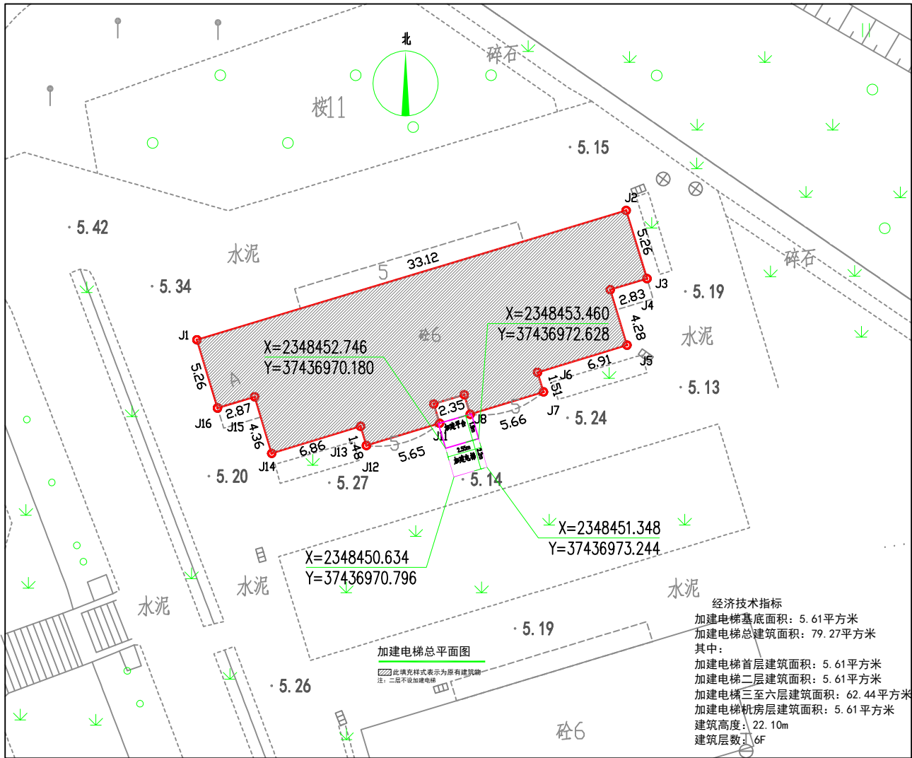
总平面图
