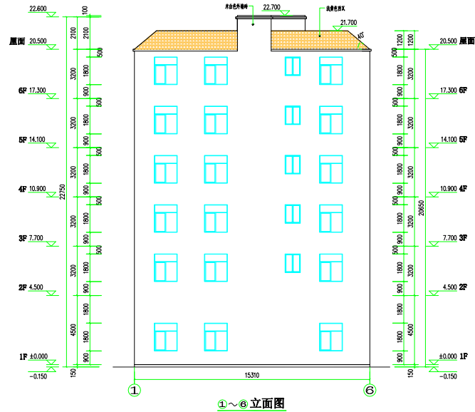
①~⑥ 立面图
