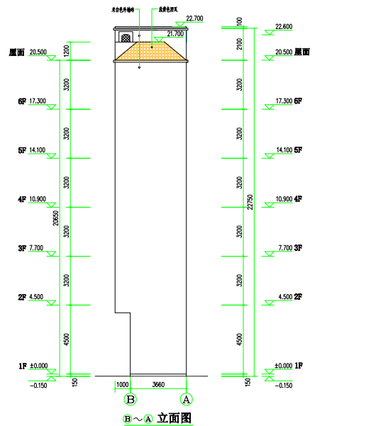
③~② 立面图
