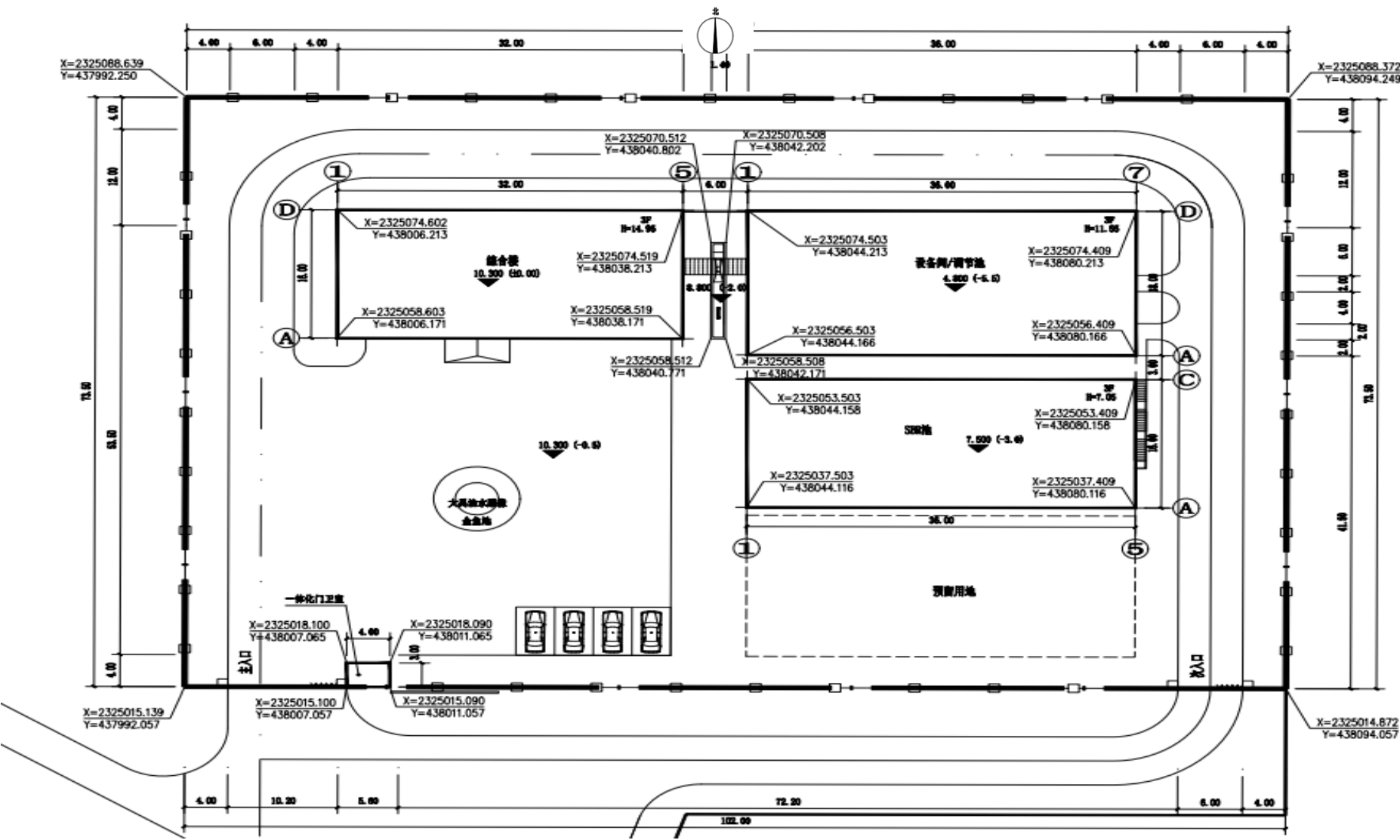
附图 1 污水处理厂厂区平面布置图
