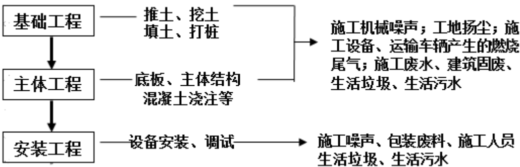
图 5-1 污水处理厂施工期工艺流程及产污环节图
