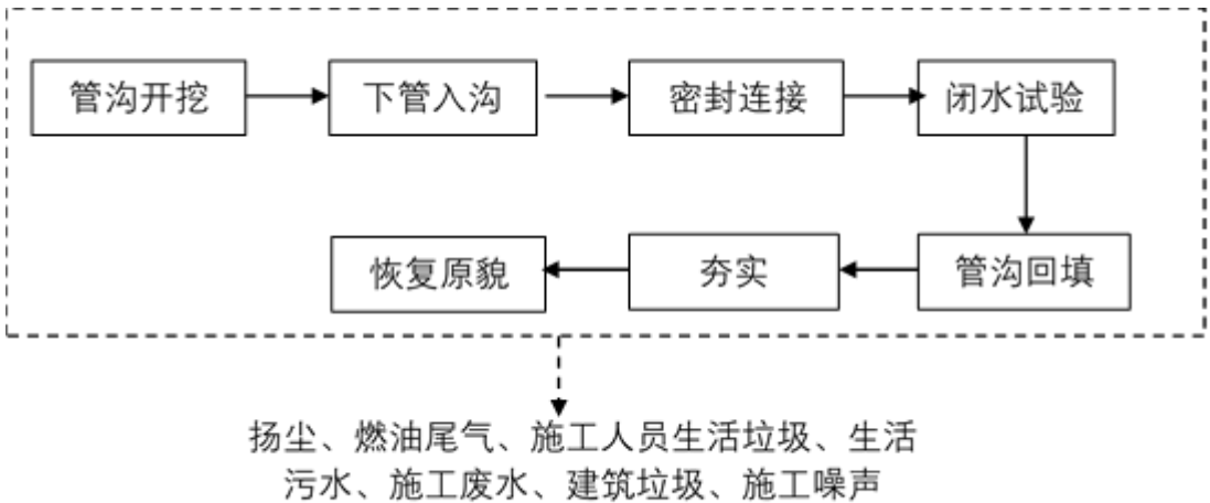
图 5-2 配套管网施工期工艺流程及产污环节图
