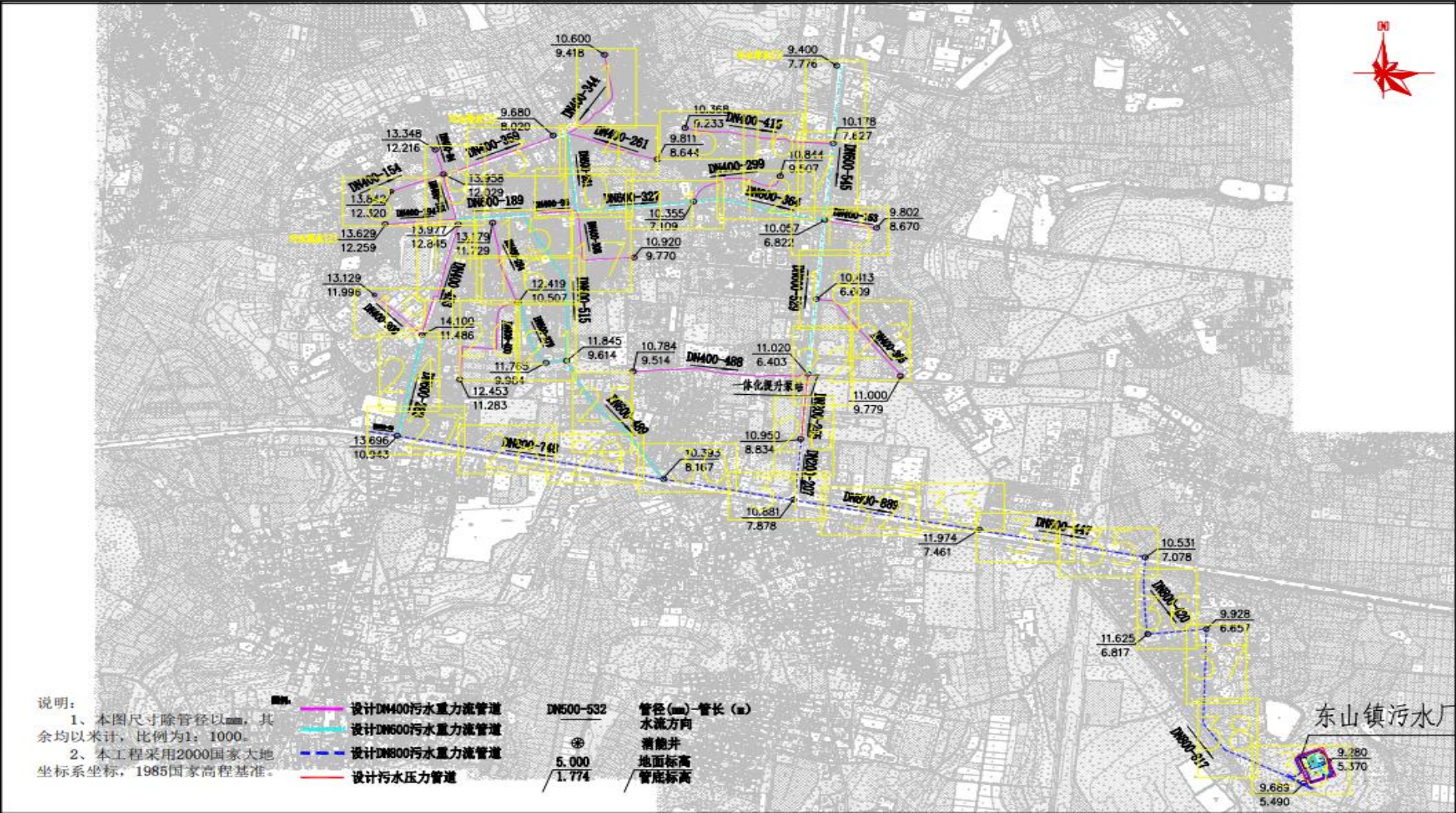
附图 4 配套管网走向分布图
