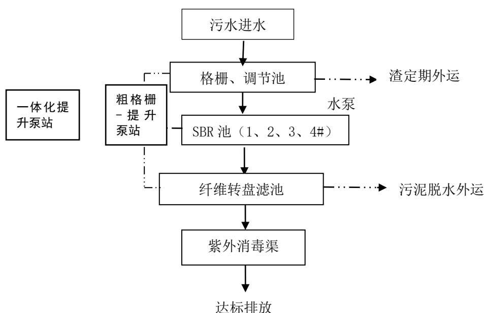
图 5-3 运营期废水处理工艺流程及产污环节图
