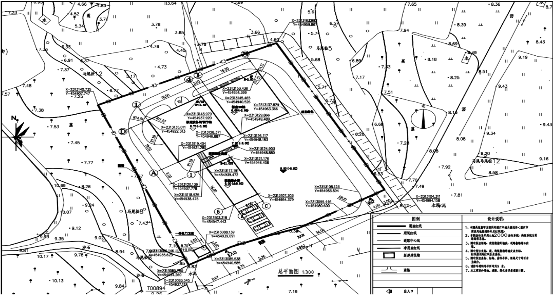
附图 3 污水处理厂厂区平面布置图
